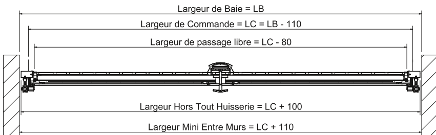
Coupe horizontale pose en tunnel OD-IL
