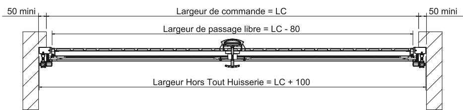
Coupe horizontale pose en applique OD-IL
